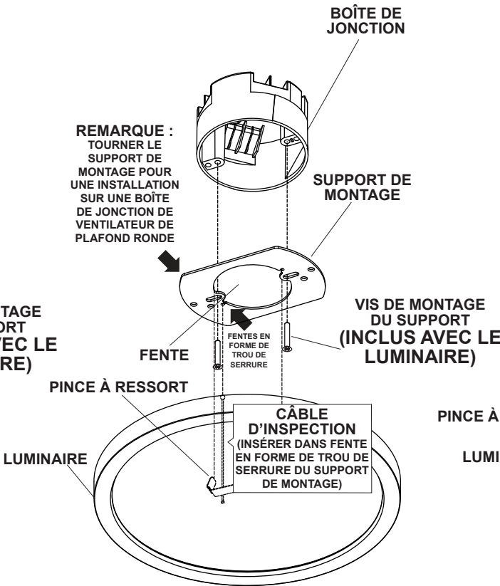
Fig. 2 INSTALLATION SUR LA BOÎTE DE JONCTION DU VENTILATEUR DE PLAFOND RONDE
